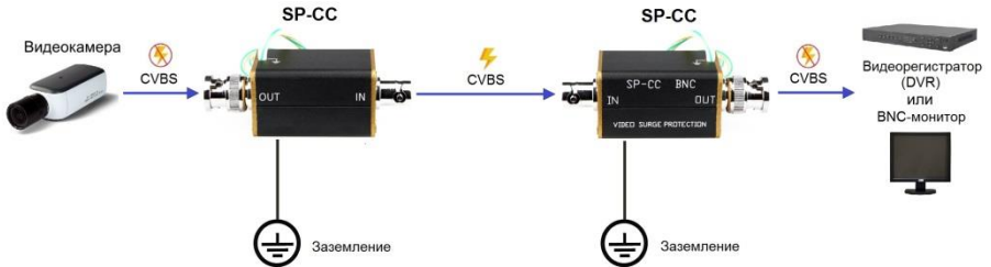
Рис.3 Схема подключения SP-CC.
