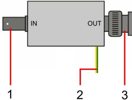
Рис.2 Разъёмы SP-CC
